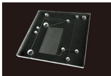
マイクロ流体デバイスサンプル
